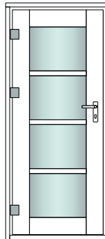
MH-ET-GV1-QS Madriers: 15mm Dim.: 84x194cm
